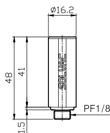
SL18
