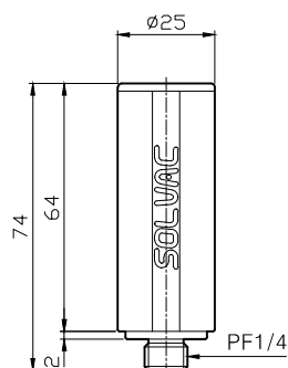
SL14W
