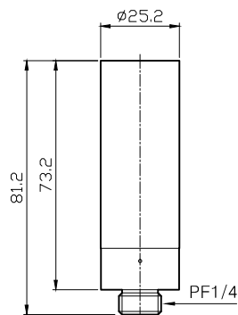
SL14W
