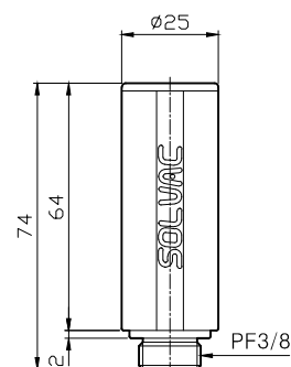
SL38W
